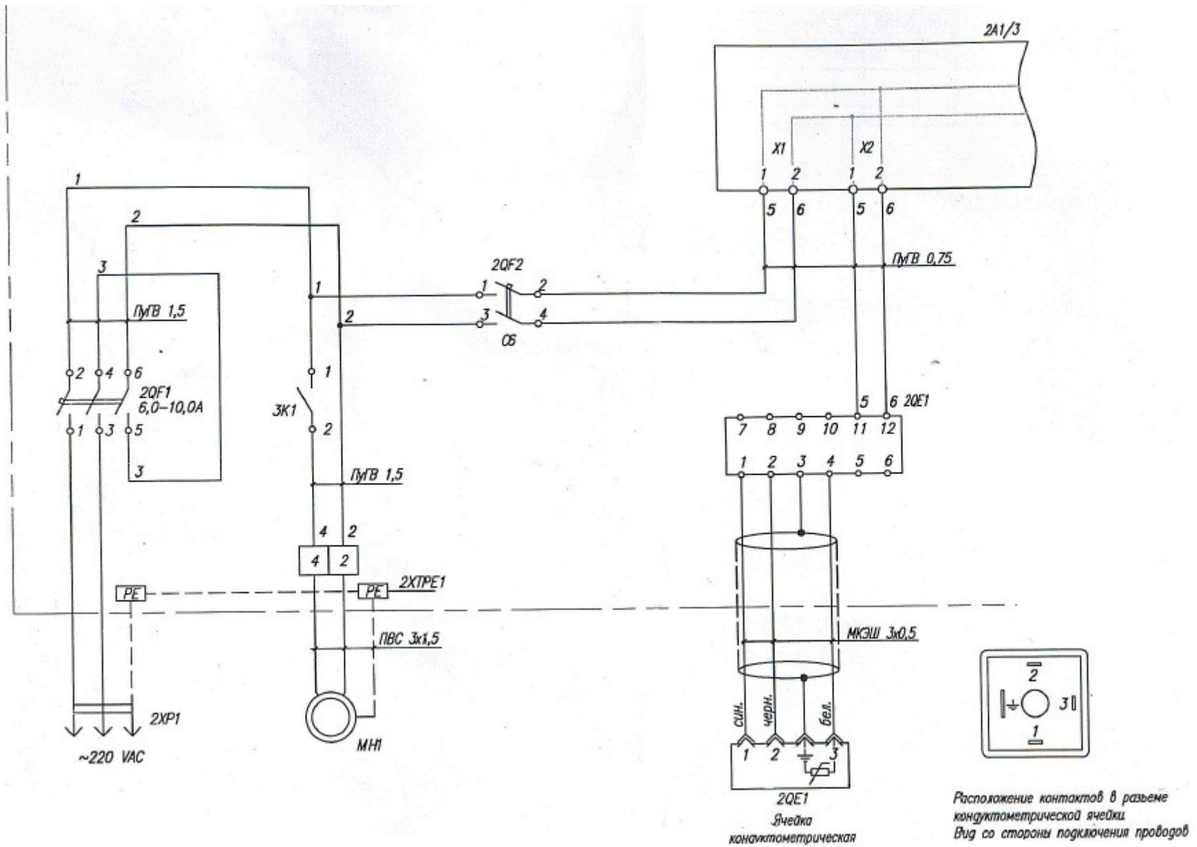
Рис 26. Принципиальная электрическая схема установки «Комплекс мембранной очистки воды 0,06...1,0 м³/ч со стандартными мембранами»*
