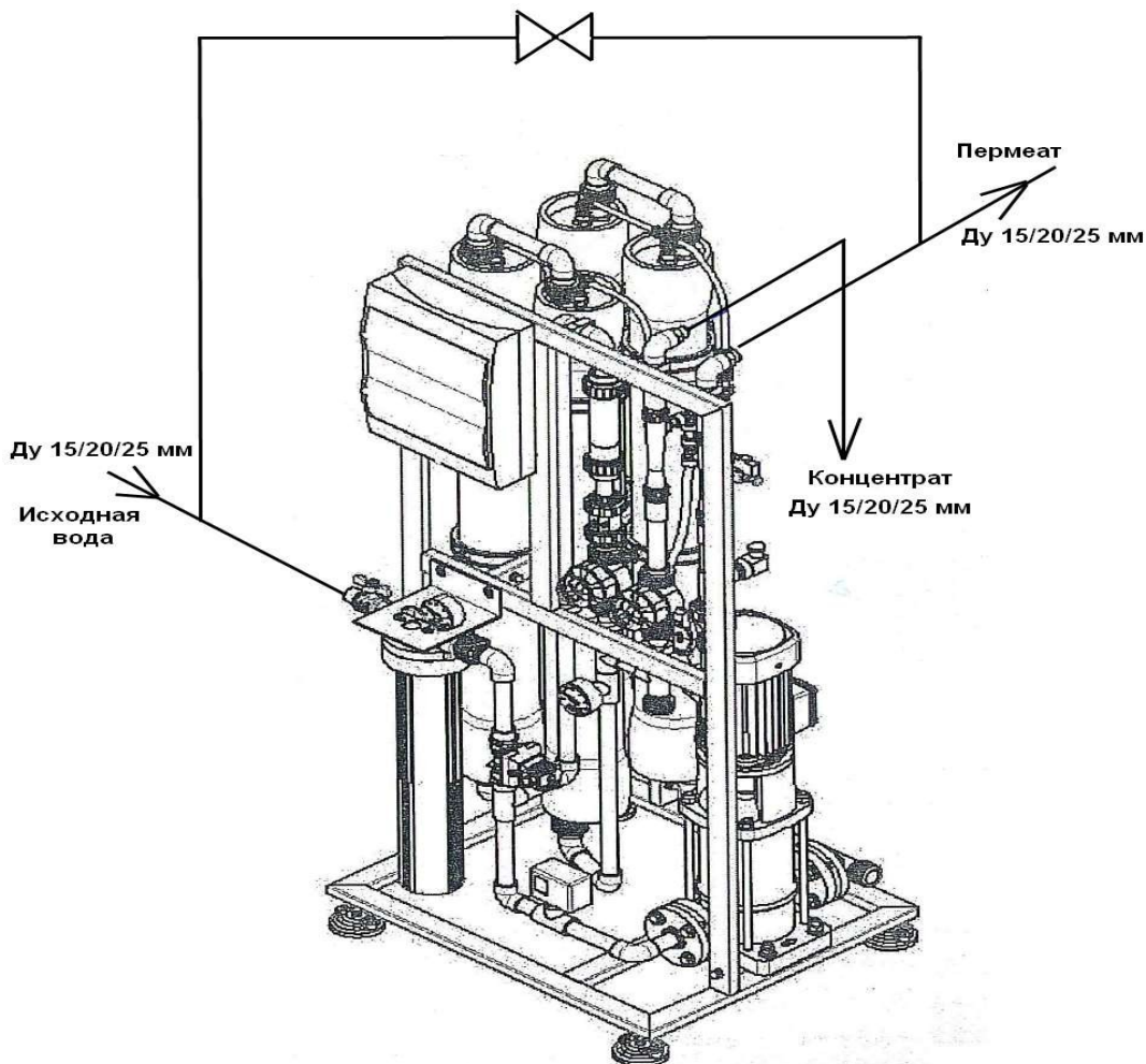
Рисунок 2 — Схема монтажа установки КМОВ 0,06-1,0 СМ
